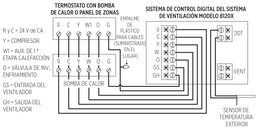
FIGURA 2: CABLEADO A LA BOMBA DE CALOR
