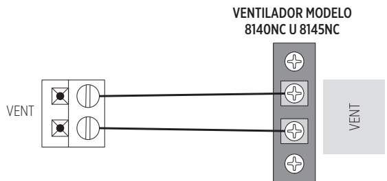
FIGURA 3: CABLEADO AL VENTILADOR DE AIRE FRESCO MODELO 8140NC U 8145NC
