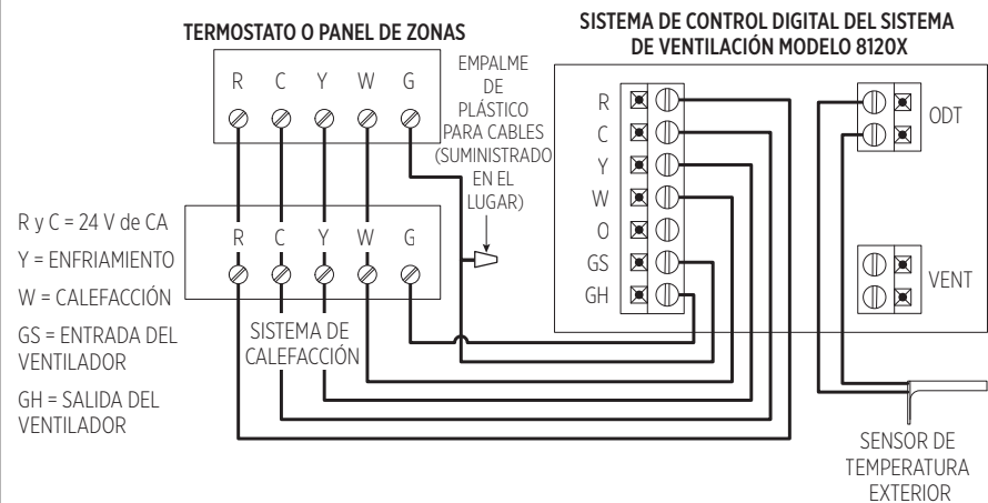
FIGURA 1: CABLEADO AL CALEFACTOR
