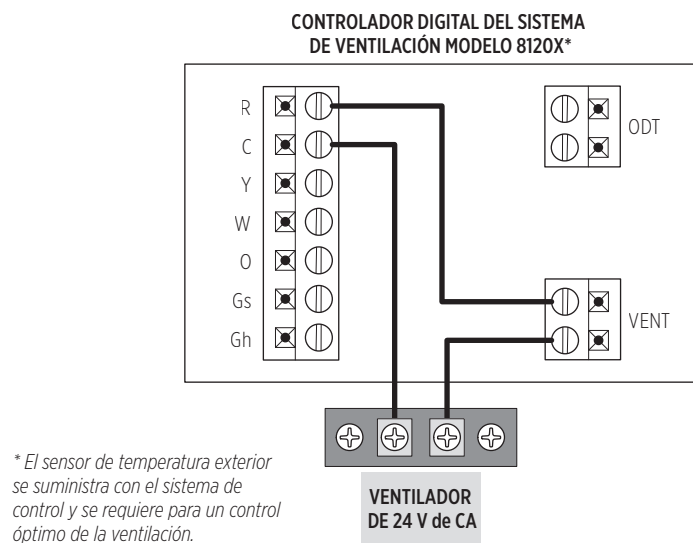
FIGURA 4: CABLEADO AL VENTILADOR DE AIRE FRESCO MODELO 8142NC
