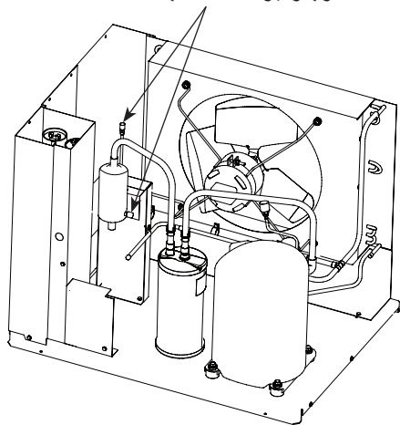
التوصيلات البديلة لصمامات شريدنر بوحدة التكتيف
