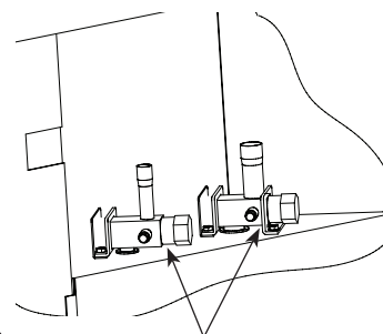
RACCORDER LA POMPE À VIDE AUX ROBINETS D'ARRÊT DES CONDUITES
