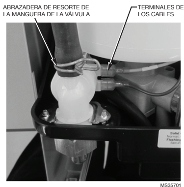
Fig. 5. Cómo desconectar la válvula de llenado existente.
