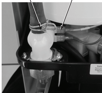
Fig. 3. Déconnexion de l'ancienne vanne de remplissage.
