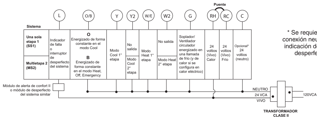
Figura 2 – Sistema de una sola etapa o multietapa (sin bomba de calor) con un solo transformador
