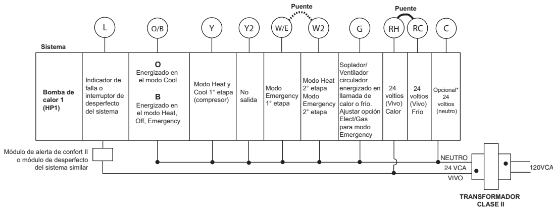
Figura 1 – Sistemas de bomba de calor
