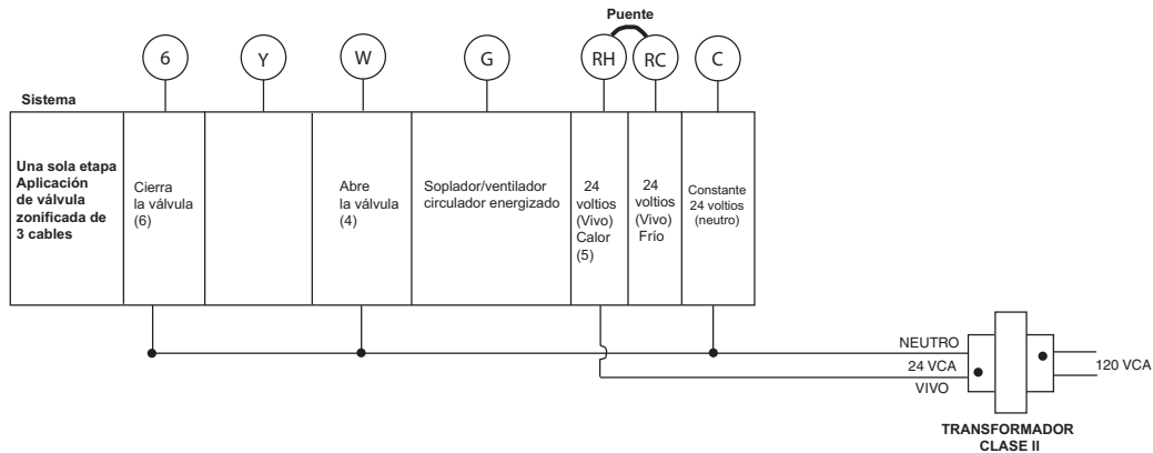
Figura 4 – Conexiones de la válvula zonificada de sólo calor de 3 cables (SPDT)
