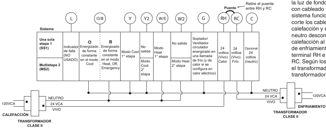
Figura 3 – Sistema de una sola etapa o multietapa (sin bomba de calor) con dos transformadores
