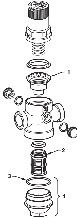
Fig. 5. Pièces de rechange.
